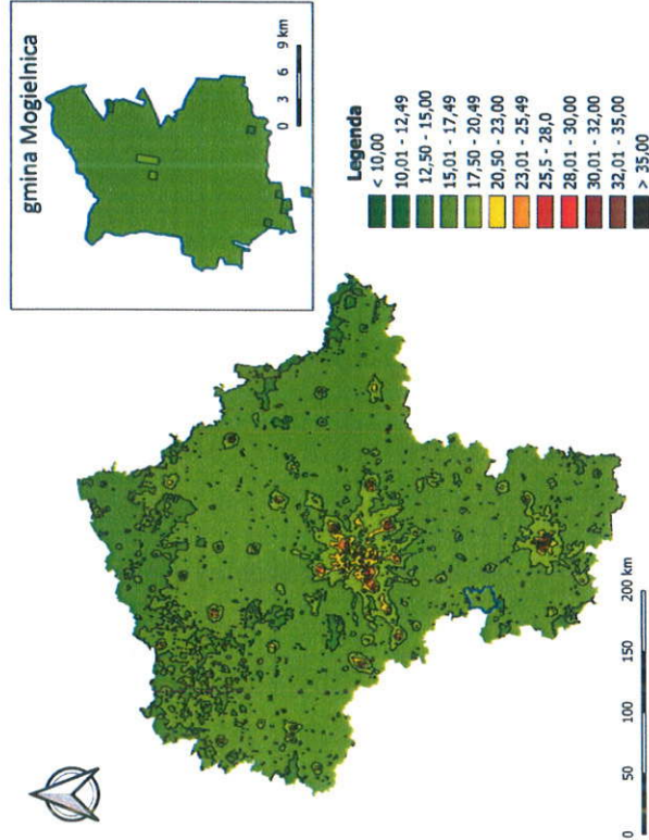
Rysunek 5. Rozkład stężeń PM 2,5 na obszarze województwa mazowieckiego i gminie Mogielnica w 2016 roku, cel: ochrona zdrowia
